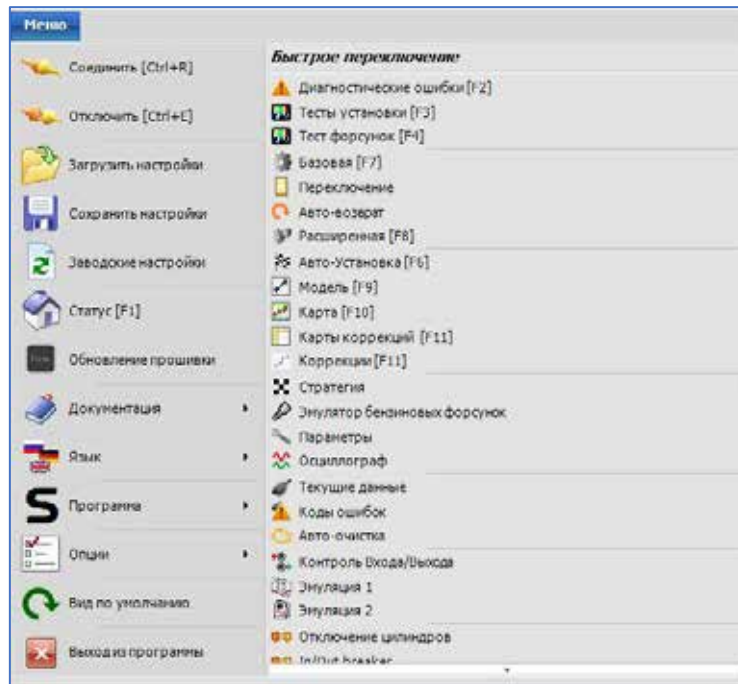
Рис. 2.15 Выпадающее меню
