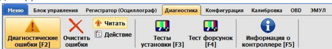
Рис. 2.36 Вкладка «Диагностика»
