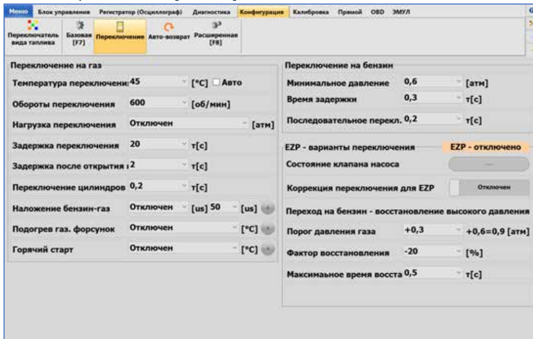
Рис. 2.56 Окно переключения
