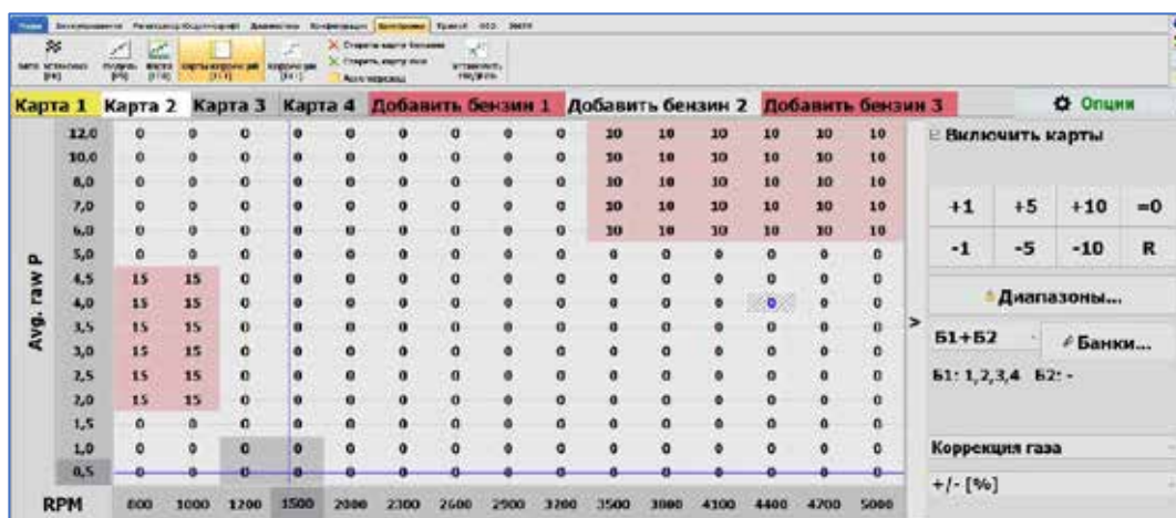
Рис. 2.80 Карты коррекций
