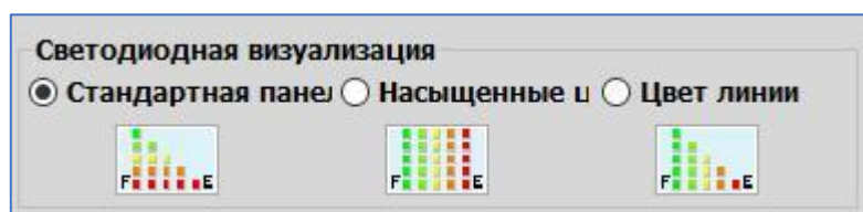
Рис. 2.50 Визуализация светодиодов
