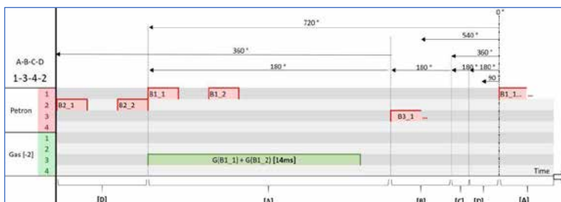
Рис. 2.119 Визуализация стратегии [-2] и углового газового сдвига
