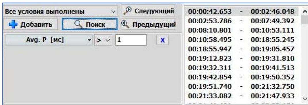
Рис. 2.33 Окно поиска
