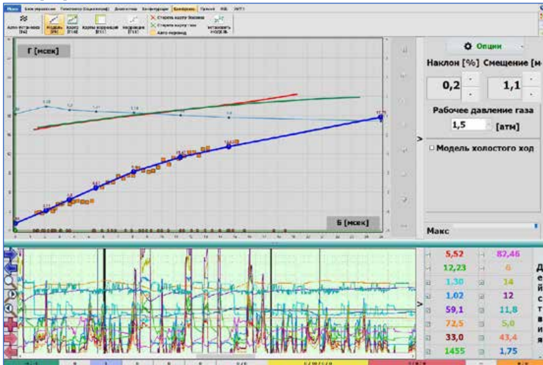
Рис. 2.71 Вкладка «Модель»
