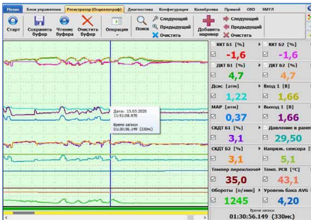
Рис. 2.31 Окно регистратора
