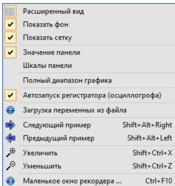
Рис. 2.32 Опции регистратора
