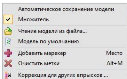
Рис. 2.73 Опции модели
