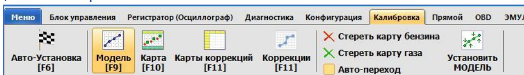
Рис. 2.61 Вкладка «Калибровка»
