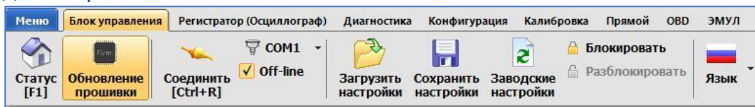
Рис. 2.22 Вкладка Контроллер
