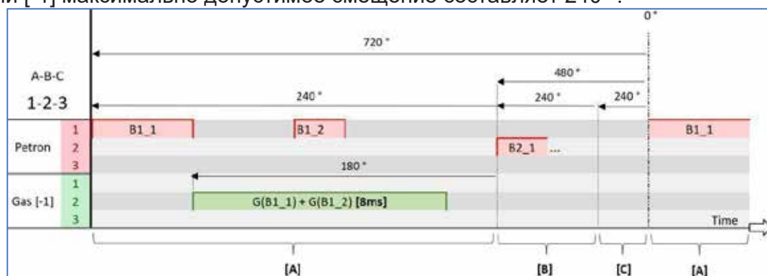
Рис. 2.121 Визуализация стратегии [-1] в трехцилиндровом двигателе с последовательностью работы цилиндров 1-2-3
