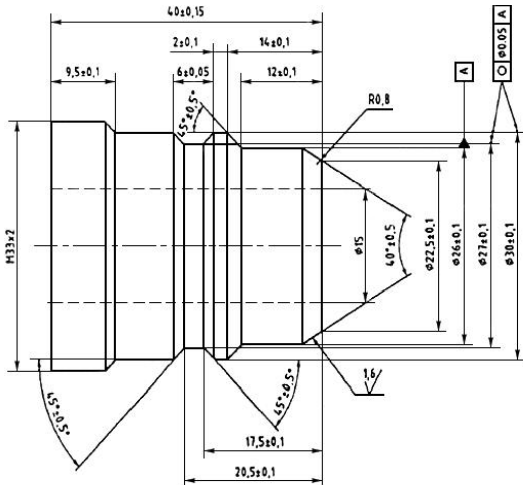
Рисунок Д.3 - Соединительный участок заправочного блока евро типа для АТС
